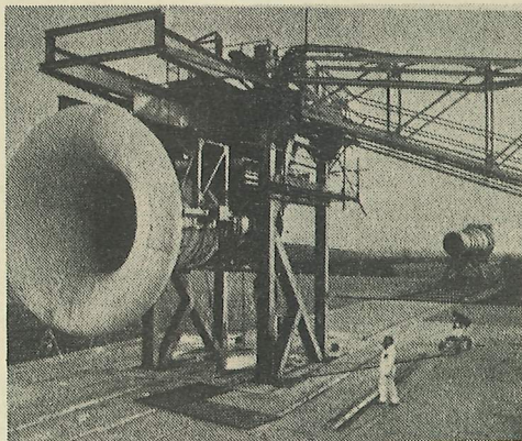
MOTOR RB-211 (PROIZVODI FIRME ROLS-ROJS) U TRENUTKU KADA SE VRŠE ISPITIVANJA NA UREĐAJIMA ZA PROCENJIVANJE BUKE.
